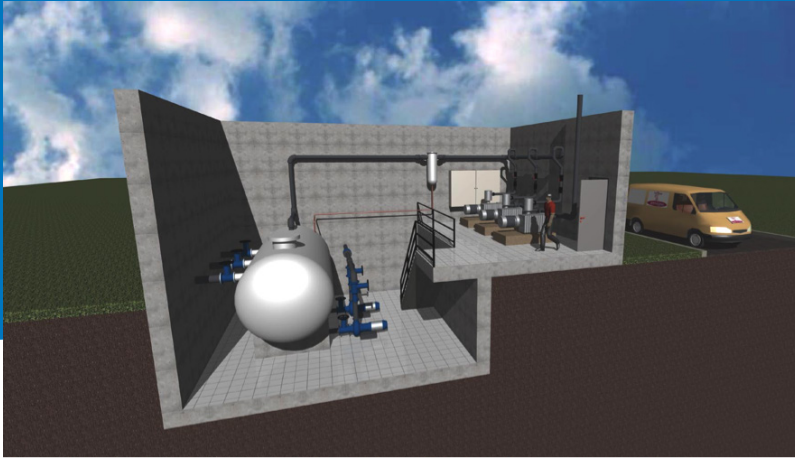
ESQUEMA DE ESTACIÓN CON BOMBAS ROTATIVAS Y TANQUE DE VACÍO EN ARQUETA SIN ENTERRAR
