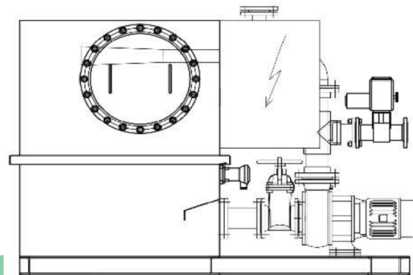
ESQUEMA DE KIT- COMPAC DE ESTACIÓN DE EYECTORES
