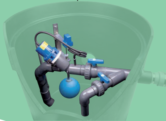
Arqueta con válvula Vacuflow® Q300
