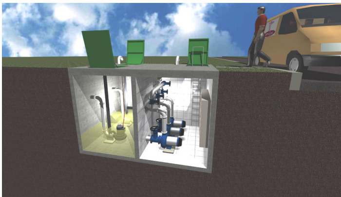
ESQUEMA ENTERRADO DE ESTACIÓN DE VACÍO POR EYECTORES
